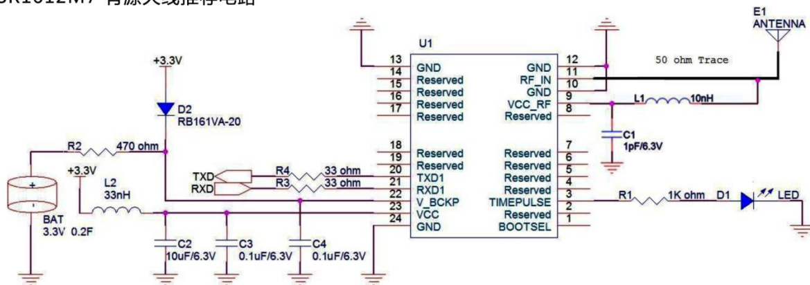
SR1612M7 有源天线推荐电路
