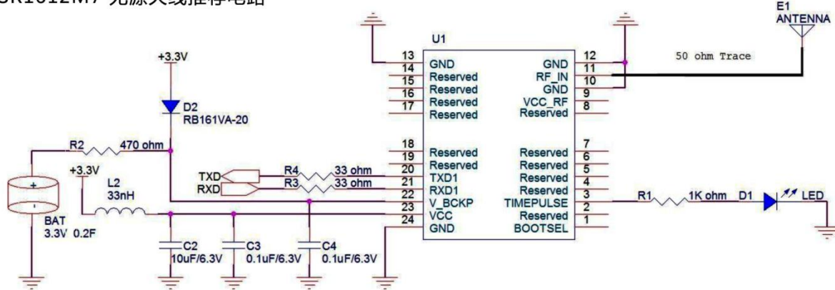
SR1612M7 无源天线推荐电路
